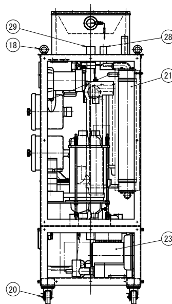
Back view 背面
