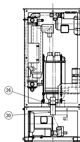
B-B section view B-B断面
